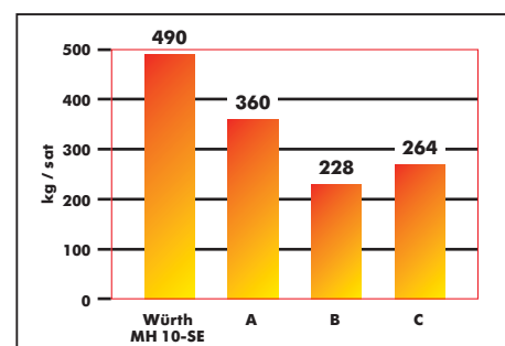
Materijal: beton B45; Smjer rada vertikalni; Alat: špic-majzl.
