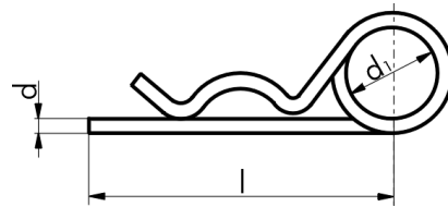
Izvedba 3: sa duplom očicom
