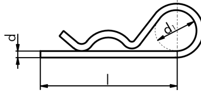
Izvedba 1: sa jednostavnom očicom
