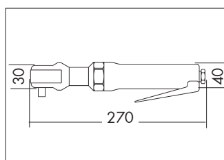
Dimenzije izvedbe 1/2"
