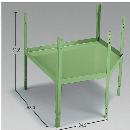
Kutna polica Art.-Nr. 0961 03 Art.-Nr. 0961 903
