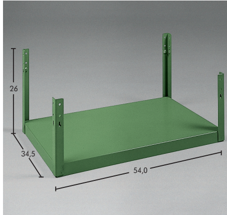
Bazna polica Art.-Nr. 0961 1 Art.-Nr. 0961 91
