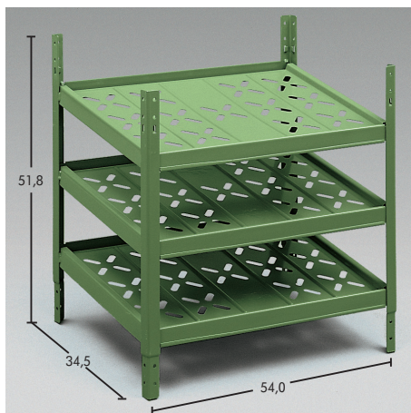
Police za velike i male kartonske dispenzere Art.-Nr. 0961 3 Art.-Nr. 0961 93
