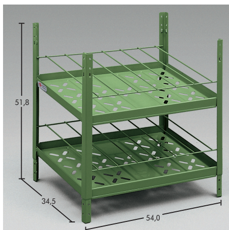
Dvostruka polica za 300-ml doze Art.-Nr. 0961 5 Art.-Nr. 0961 95
