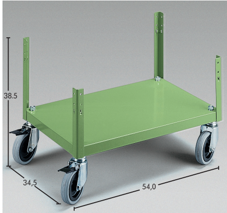
Bazna polica na točkovima Art.-Nr. 0961 01 Art.-Nr. 0961 901 1
