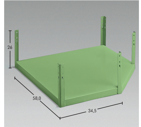
Kutna bazna polica Art.-Nr. 0961 02 Art.-Nr. 0961 902
