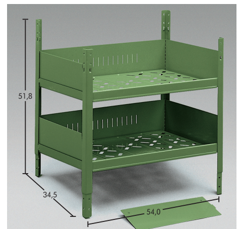
Dvostruka polica otvorena Art.-Nr. 0961 50 Art.-Nr. 0961 950
