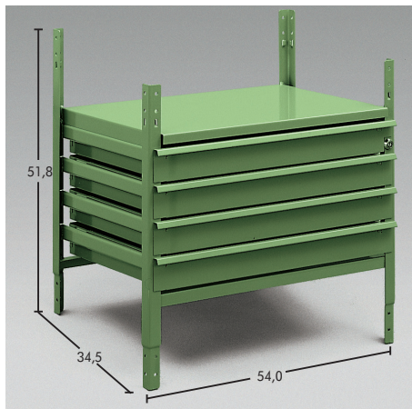
Ladice za setove Art.-Nr. 0961 2 Art.-Nr. 0961 92
