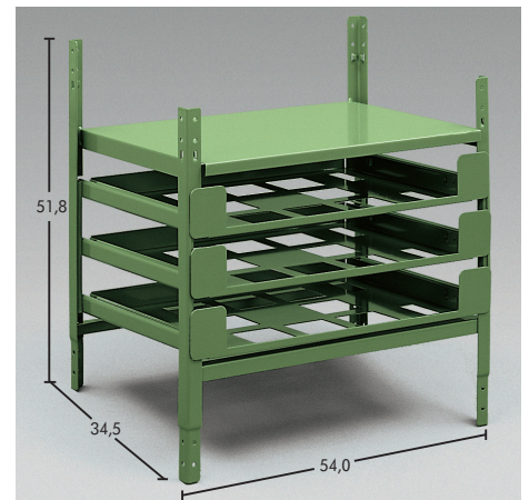
Ladice za ORSY 200 setove Art.-Nr. 0961 200 Art.-Nr. 0961 920 0
