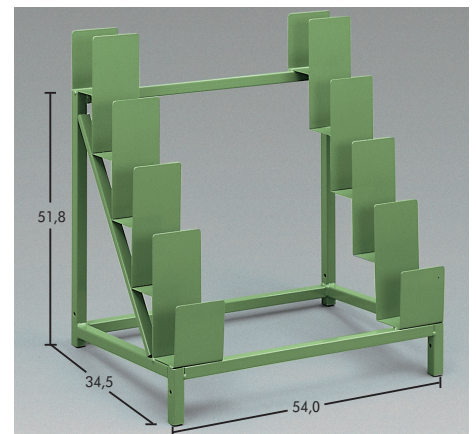
Police za navojne šipke Art.-Nr. 0961 9 Art.-Nr. 0961 99
