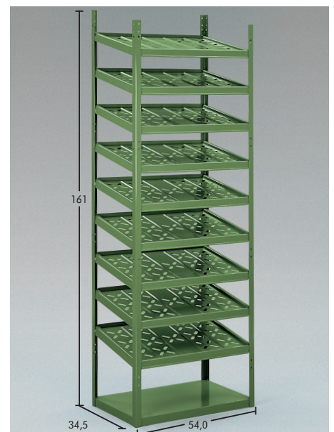
Police za ORSY velike i male kartonske kutije Art.-Nr. 0961 13 Art.-Nr. 0961 913
