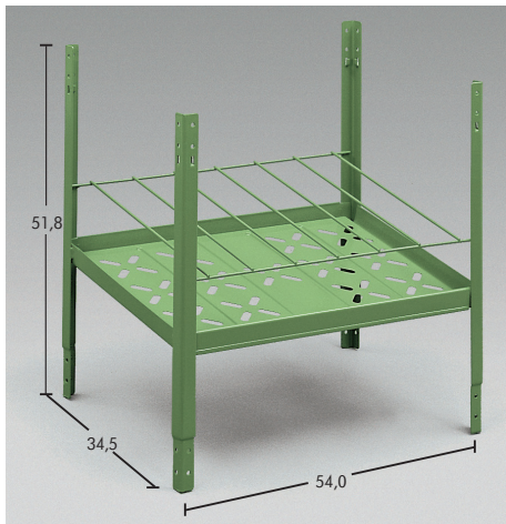
Polica za 500-ml doze Art.-Nr. 961 17 Art.-Nr. 961 97
