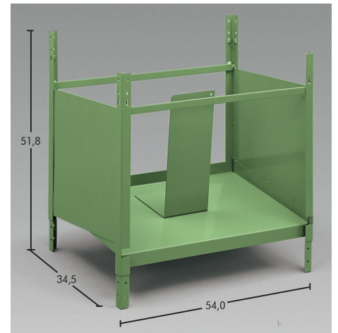
Polica za brzo-ugradive nosače reg. tablica Art.-Nr. 961 44 Art.-Nr. 961 944
