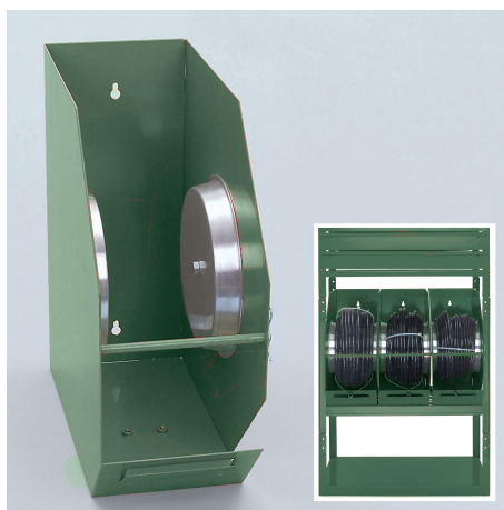
Umetak uređaja za namotavanje za poliamidske cijevi ● odgovara za ORSY u spoju sa policom 0961 4 ● moguće maksimalno 3 umetka po polici Art.-Nr. 0961 885 01 Art.-Nr. 0961 988 501
