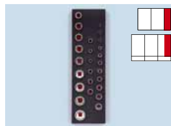
3/8" + 1/4" komplet nasadnih ključeva, 26-dijelni Art.-Nr. 0965 900 905
