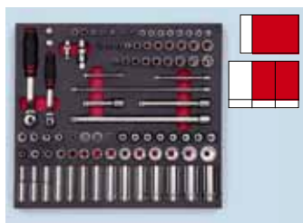
3/8" + 1/4" komplet nasadnih ključeva, 49-dijelni Art.-Nr. 0965 900 903
