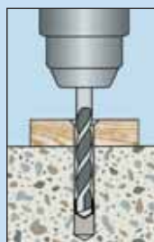
Izbušiti rupu
