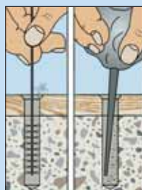
Očistiti rupu
