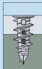
Tiplu zavrtnuti dok ne uđe u odlogu
