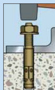
Postaviti anker zakucavanjem
