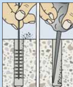
Očistiti rupu
