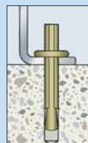
Umetnuti tiplu
