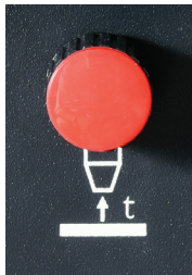
Burn-back funkcija onemogućava stvaranje kuglice na vrhu žice
